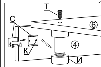
Схема крепления опоры и цоколя
